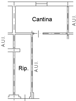
PIANTA PIANO INTERRATO H= 2.55 ml.
